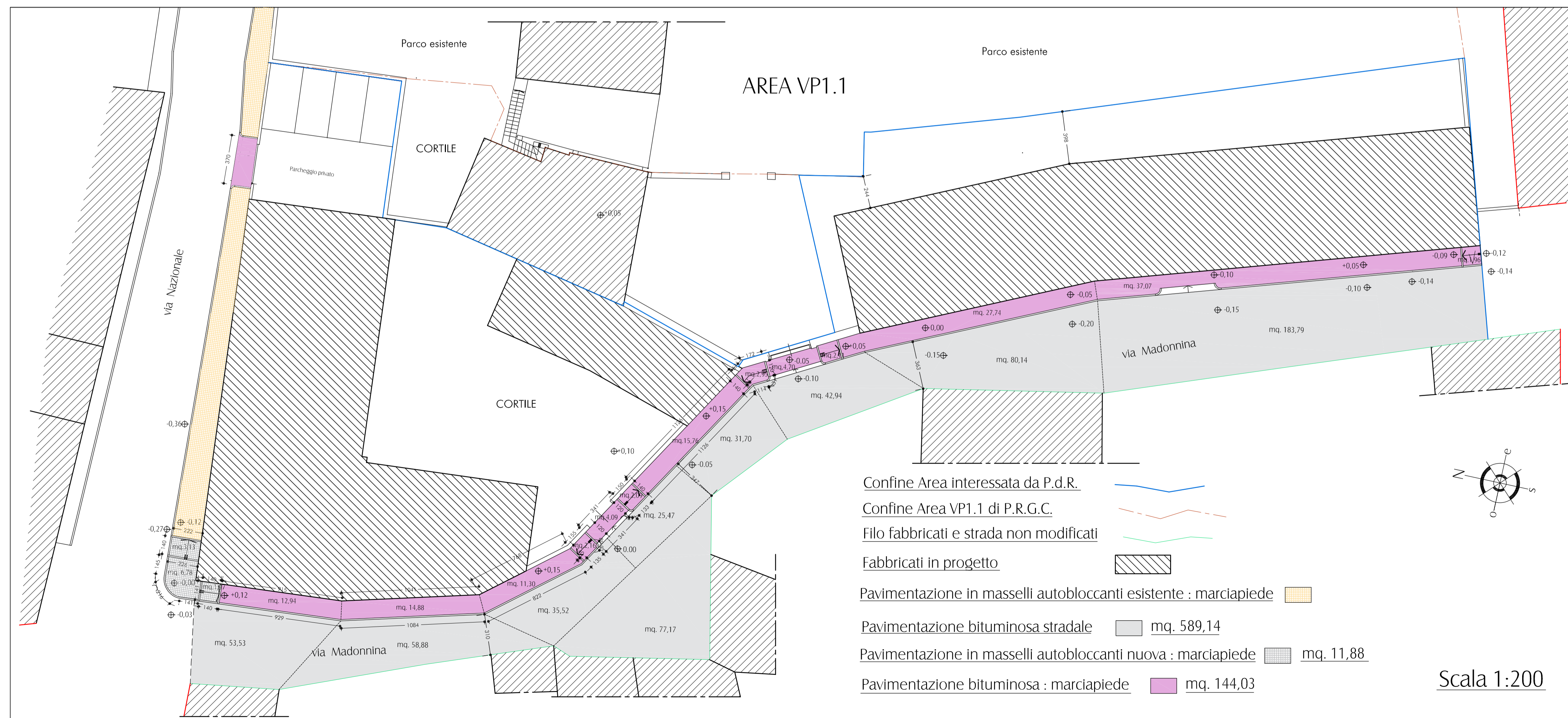
PLANIMETRIA N°8
