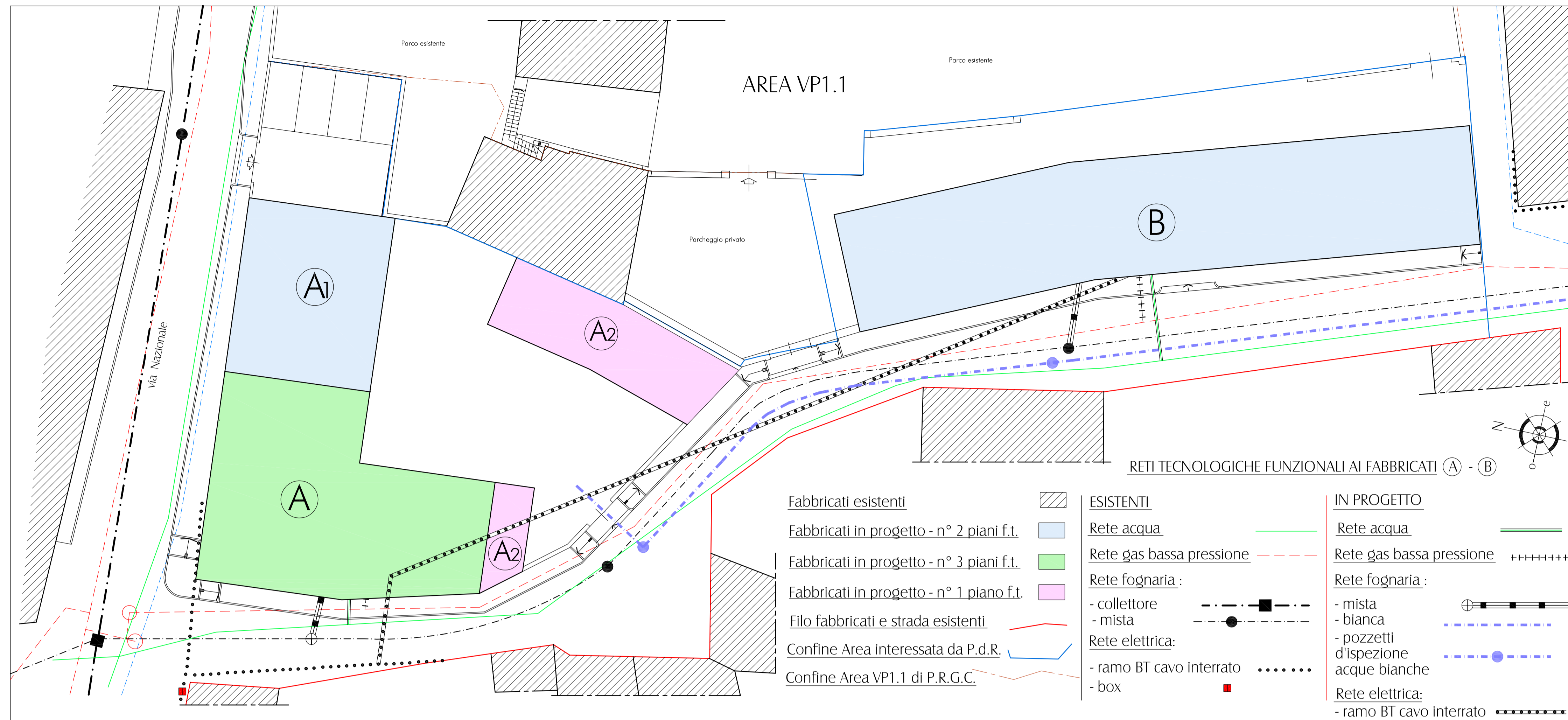
PLANIMETRIA N°7
