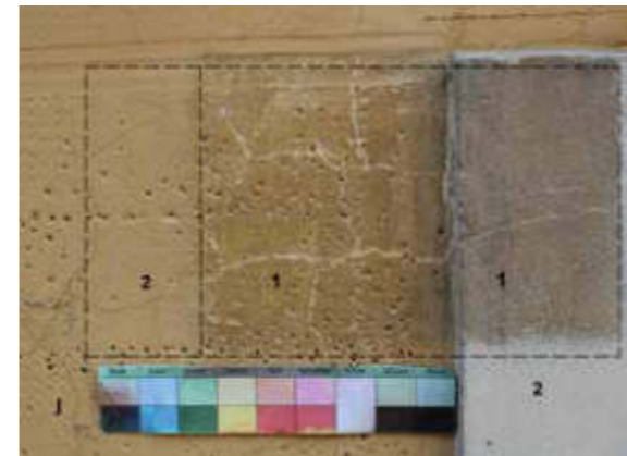
STRATIGRAFIA I
